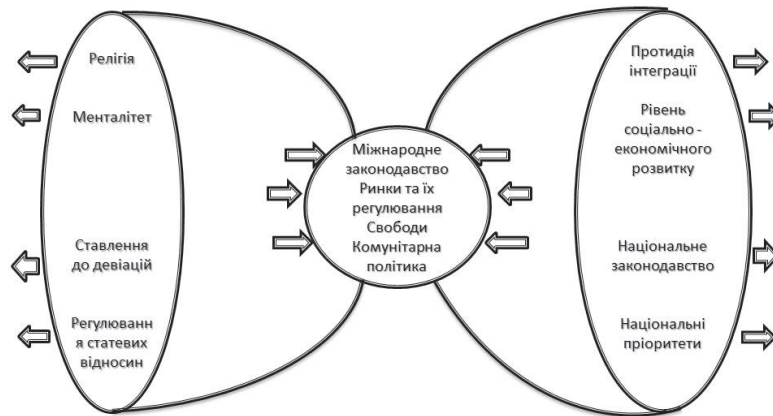
Рис. 1. Факторна модель динаміки інтеграційних відносин у країнах ЄС
